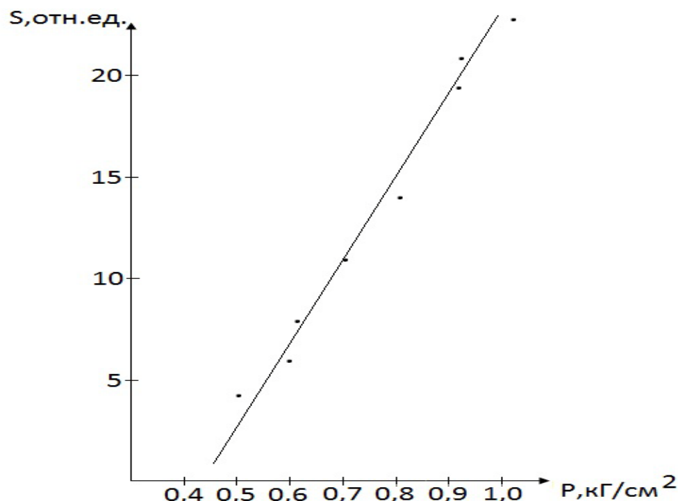
Рисунок 1 – Зависимость светочувствительности тонких слоев \text{SnI}_2 от давления воздуха
