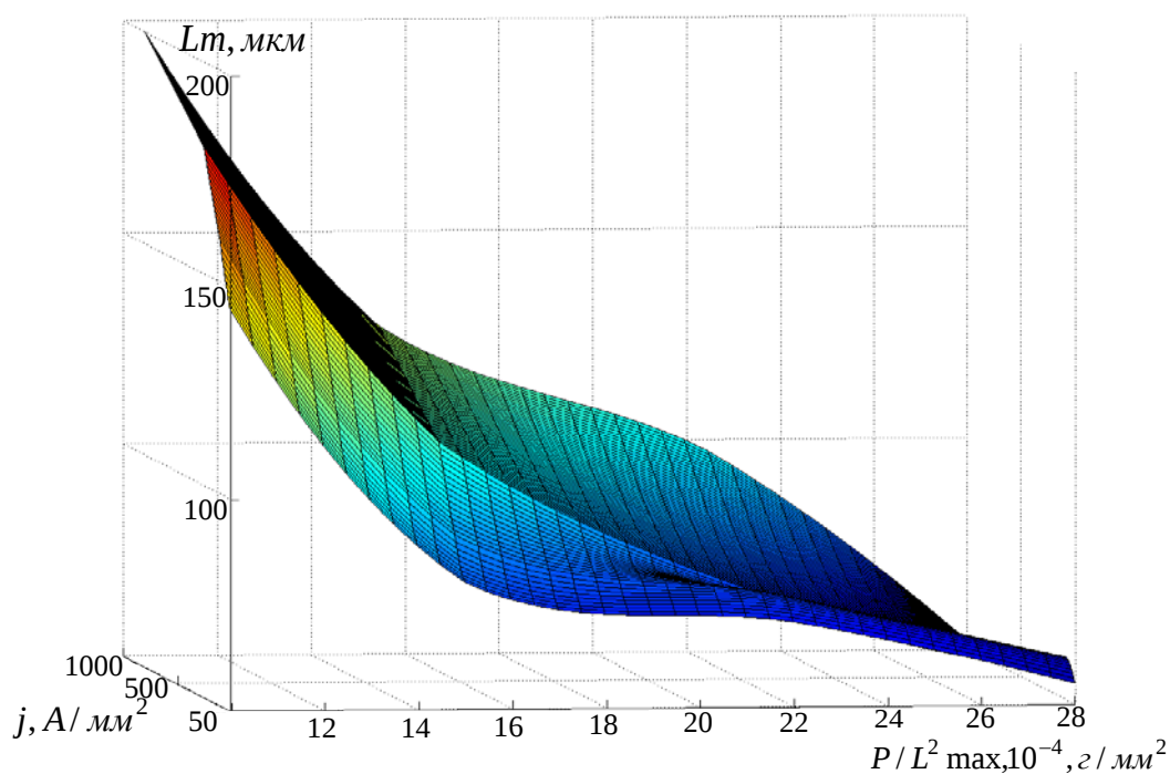
Рисунок 6 – Зависимость величины P/L^2 max от плотности тока в кристаллах висмута Вї 99,99%
