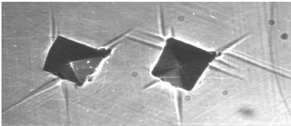
Отпечаток слева получен при нагрузке на индентор 10 г. Отпечаток справа – при той же нагрузке на индентор, но во время деформации через кристалл пропусклся импульс тока плотностью 600 А/мм 2 (х 530).
