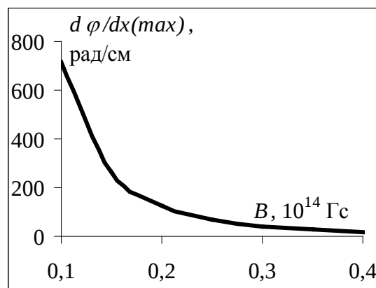
Рисунок 2 – Величина угла поворота вблизи резонанса в зависимости от B ( p_z = 0 , n_e = 10^{22} \text{ см}^{-3} , \beta = 0 )
