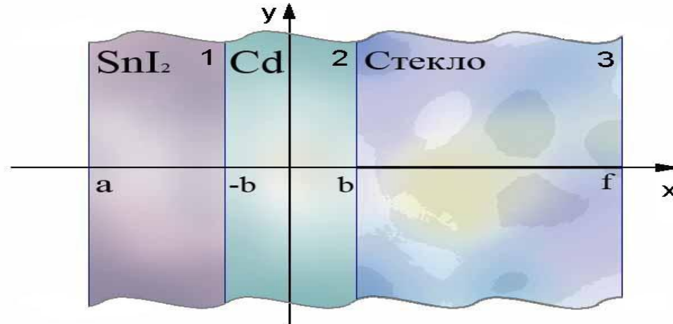
Рисунок 8 – Структура ПМД
