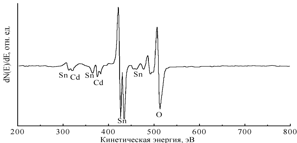
Рисунок 6 – Оже-спектр поверхности облученной структуры SnI 2 -Cd-стекло после ионного травления приповерхностного слоя
