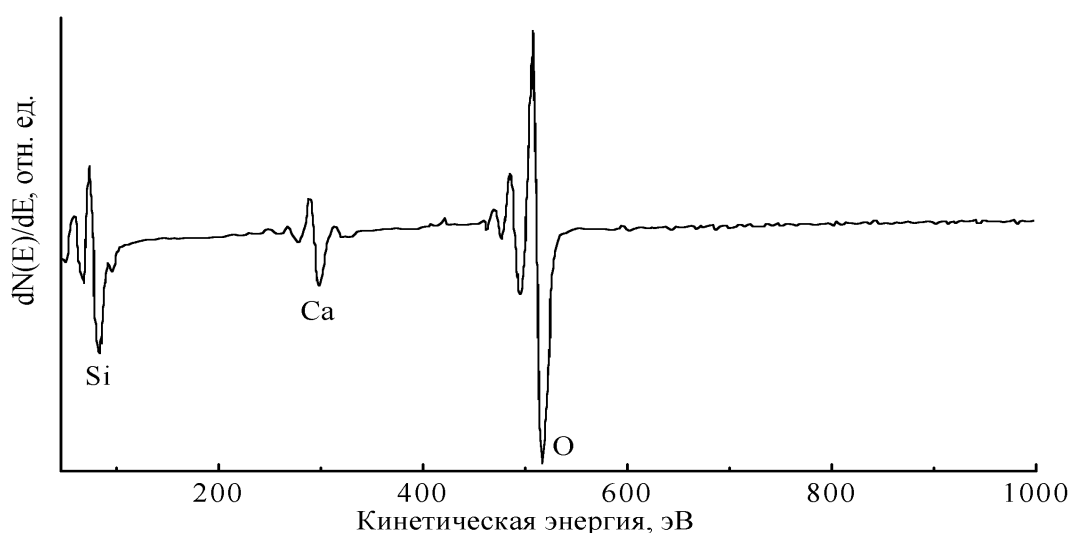
Рисунок 3 – Оже-спектр стеклянной подложки структуры после ионного травления слоев полупроводника и металла
