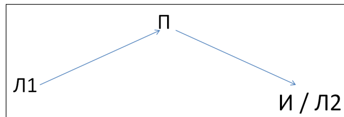
Рисунок 4. – Вариант 3 минимальной ЛП-системы (имущественной)
