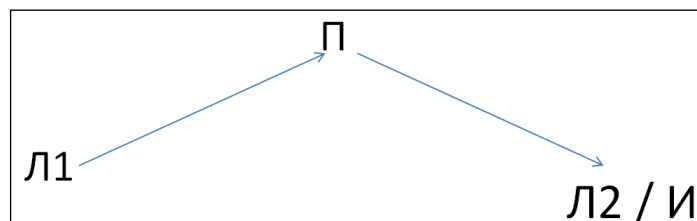
Рисунок 5. – Вариант 4 минимальной ЛП-системы (имущественной)
