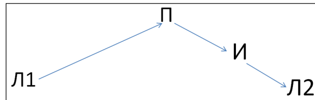
Рисунок 3. – Вариант 2 минимальной ЛП-системы (имущественной)
