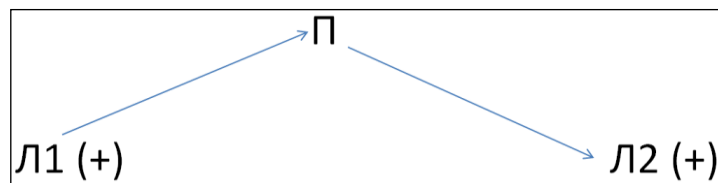
Рисунок 6. – Положительная минимальная ЛП-система
