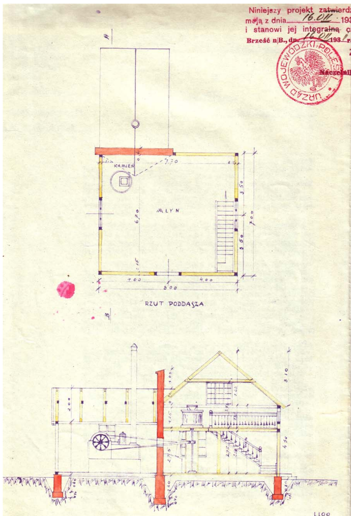
Рисунок 1. – План мельницы
