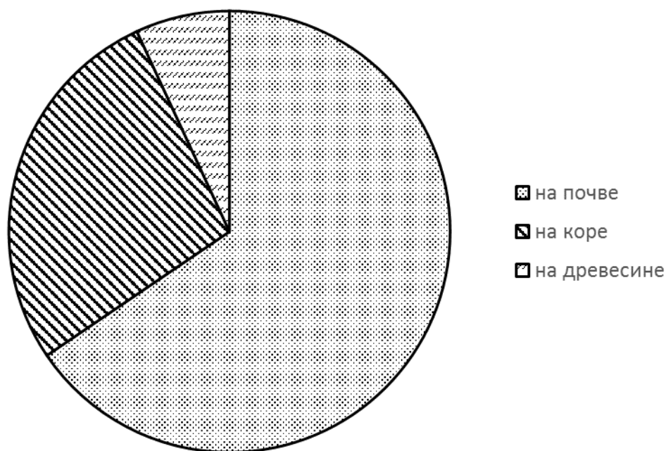
Рисунок 3. – Субстратная приуроченность Cladonia merochlororphaea в Беларуси
