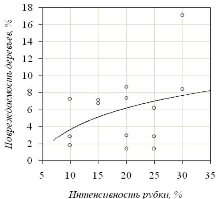
Рисунок 2 – Зависимость повреждаемости оставляемой части деревьев от интенсивности рубки
